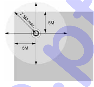
Distância máxima para evitar espaços sem cobertura
