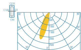
Distribuição assimétrica para iluminância vertical elevada
